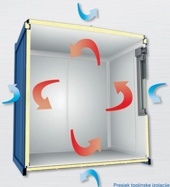
Presjek toplinske izolacije
